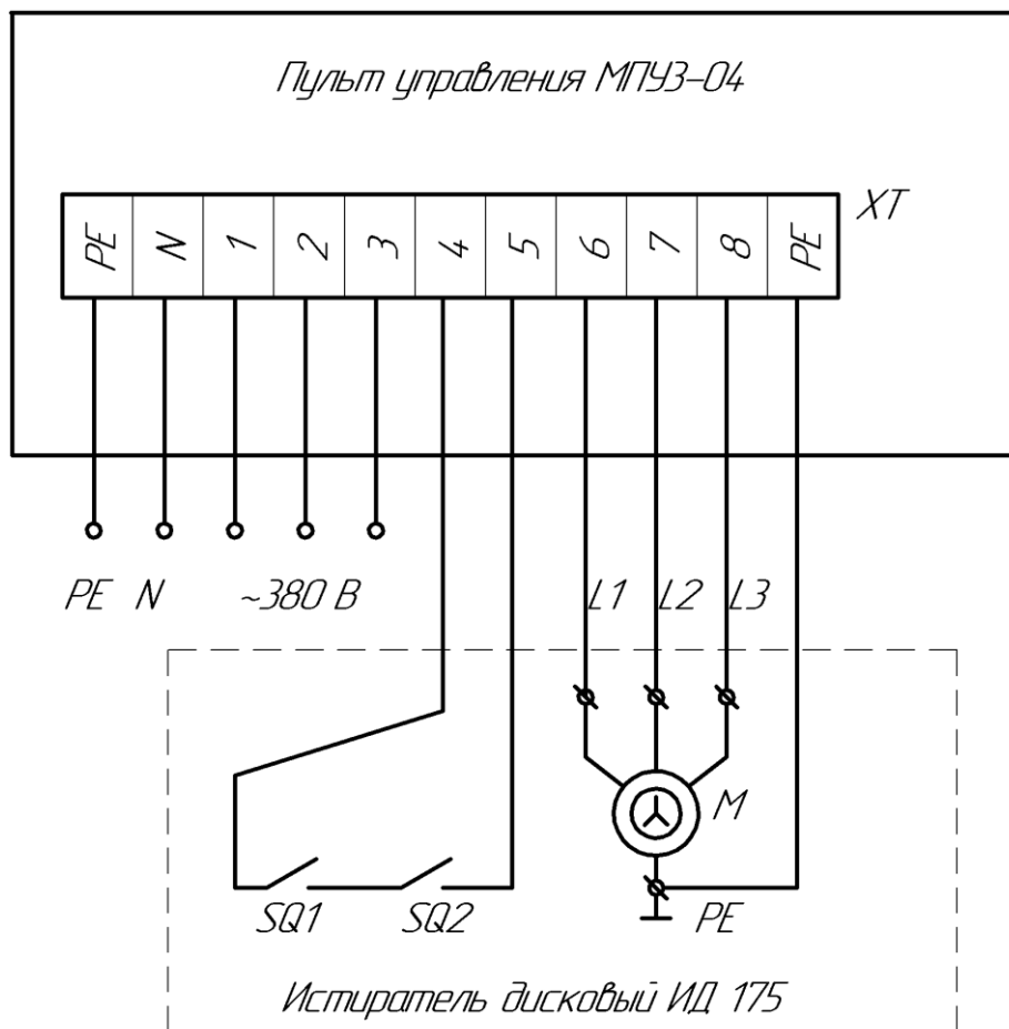
Рис. 5. Принципиальная электрическая схема
