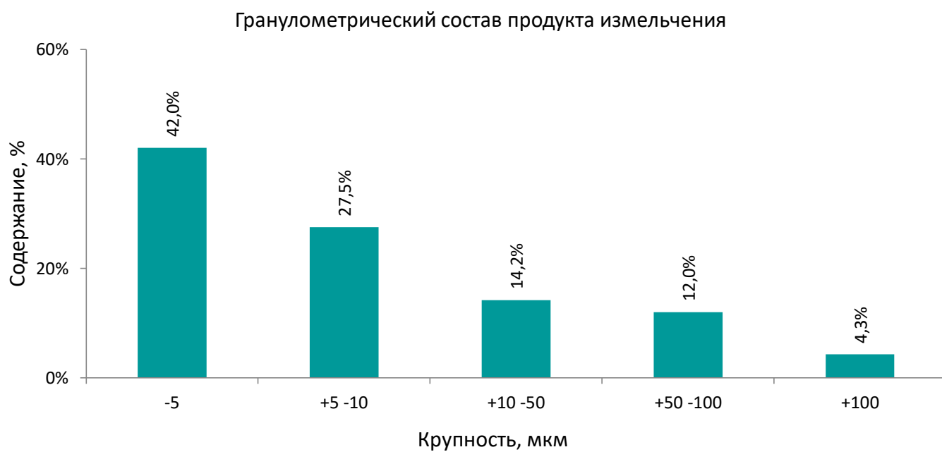
Рис. 5. Гранулометрический состав продукта измельчения
