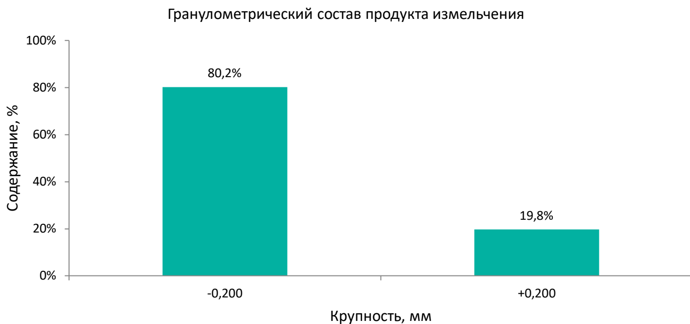
Рис. 5. Гранулометрического состав продукта измельчения
