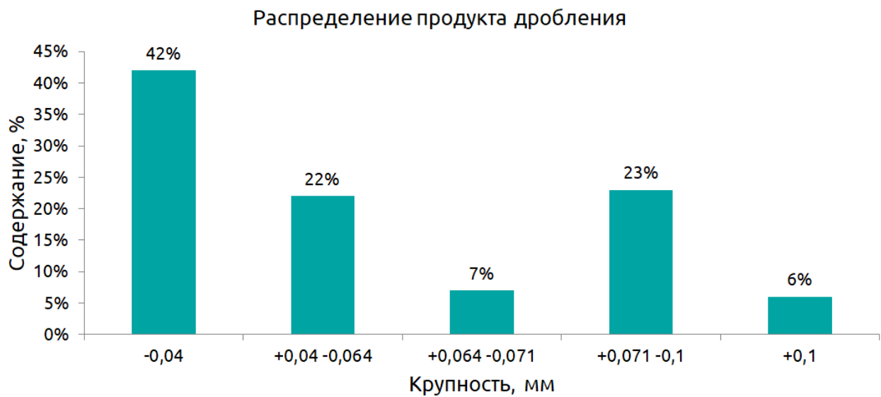
Рис. 5. Распределение продукта измельчения
