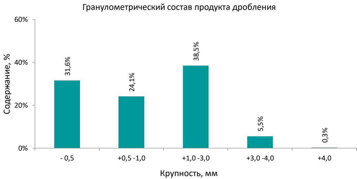
Рис. 5. Гранулометрический состав продукта дробления
