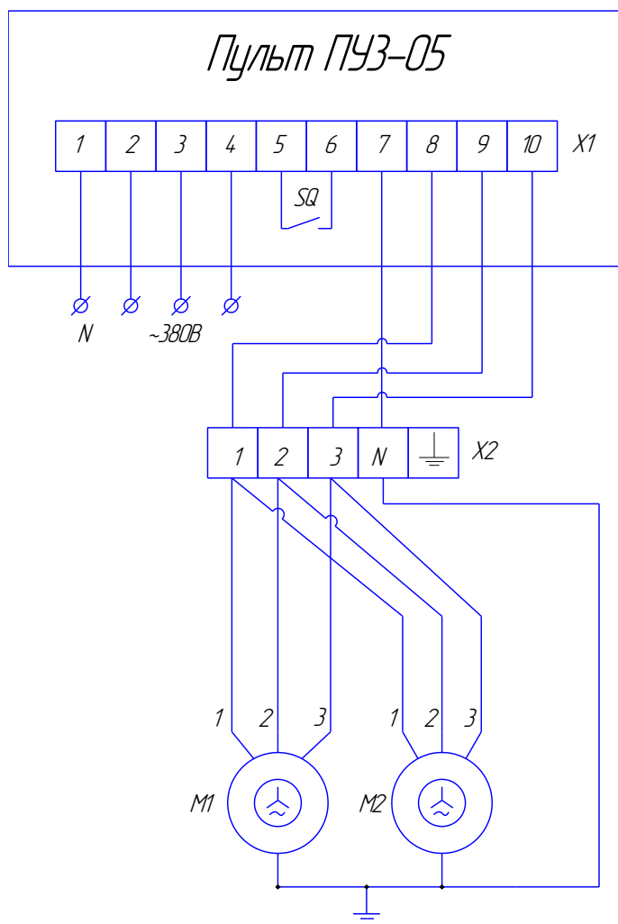
Рис.5 Принципиальная электрическая схема валковой дробилки
