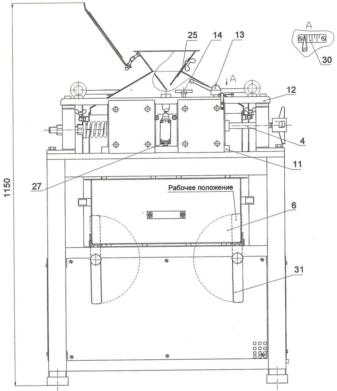
Рис 2. Вид спереди.
