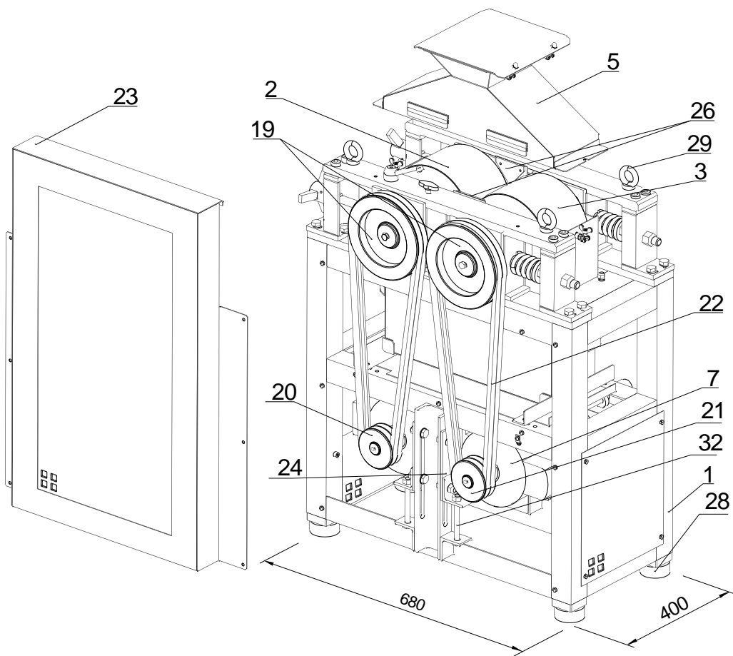
Рис 1. Вид общий.
