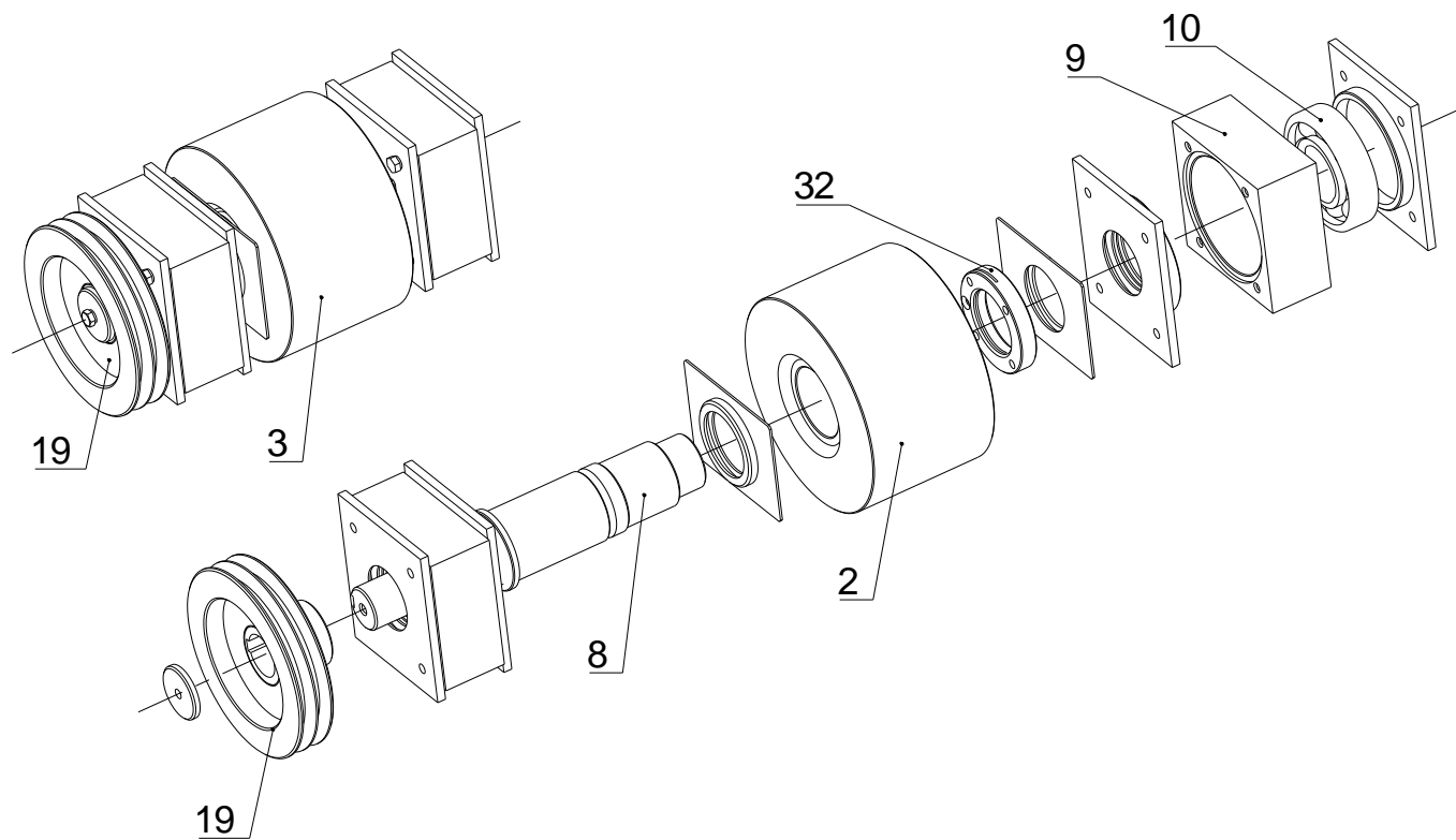
Рис 3. Валок.
