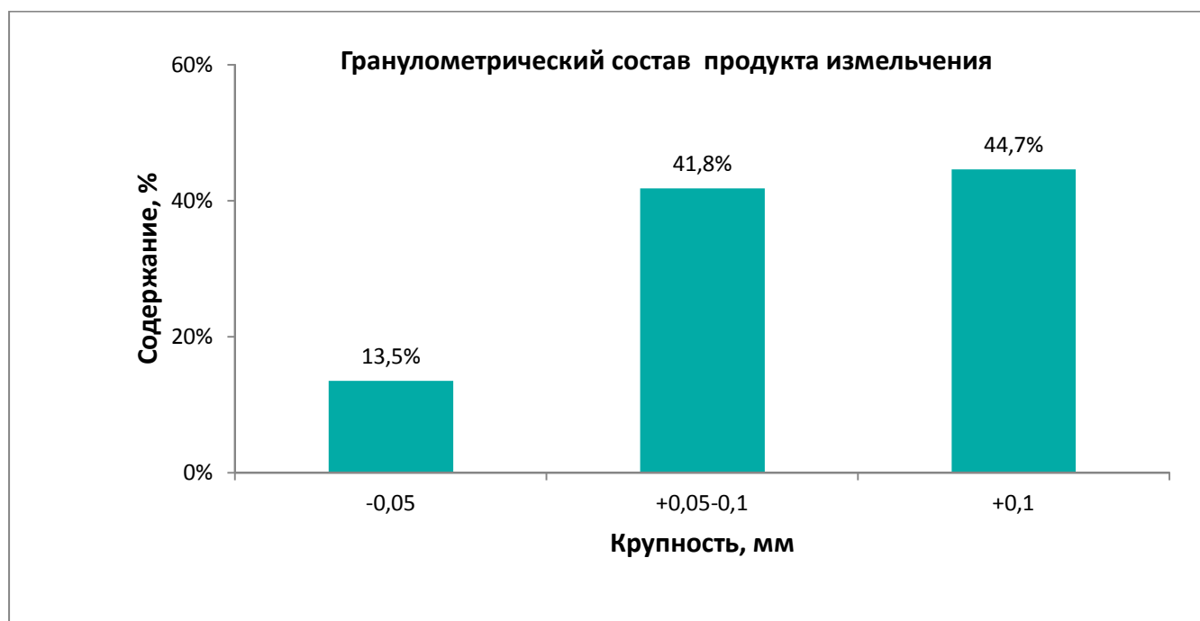
Рис. 5. Распределение продукта измельчения
