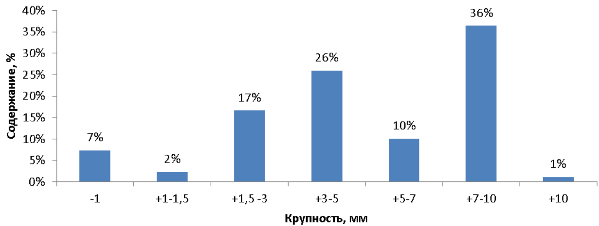
Рис. 7 Распределение продукта дробления по п. 2.1
