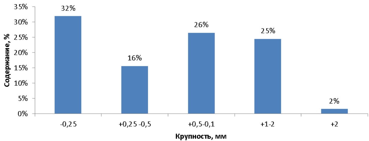
Рис. 8 распределение продукта дробления по п. 2.3
