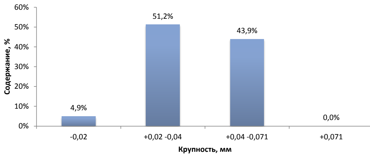
Рис. 5 Распределение продукта измельчения
